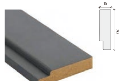
직각 2계단 (대) 2,400×70×15
